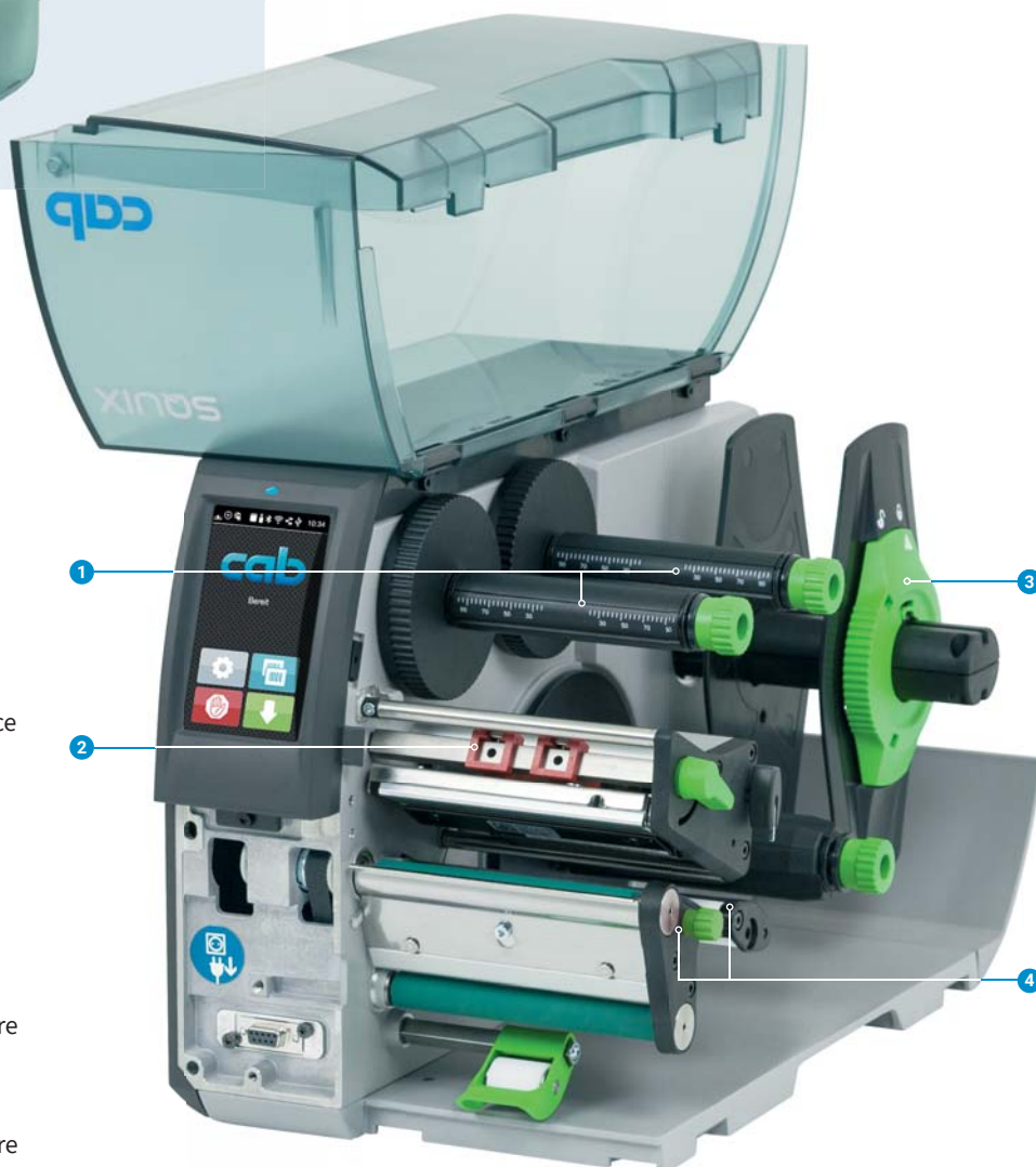
Imprimante d'étiquettes SQUIX 4 MP, modèle P avec enrouleur interne
